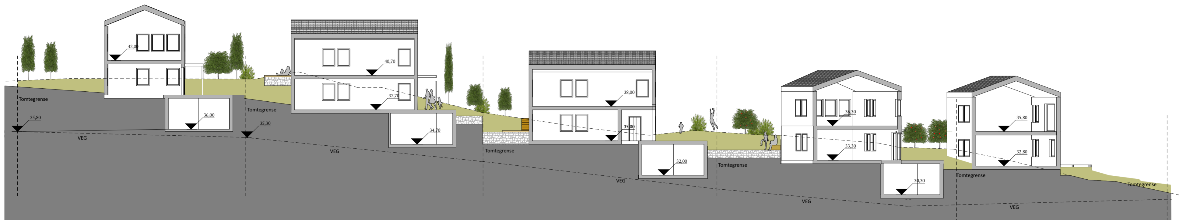
Snitt I-I gjennom felt B A2 1:200
