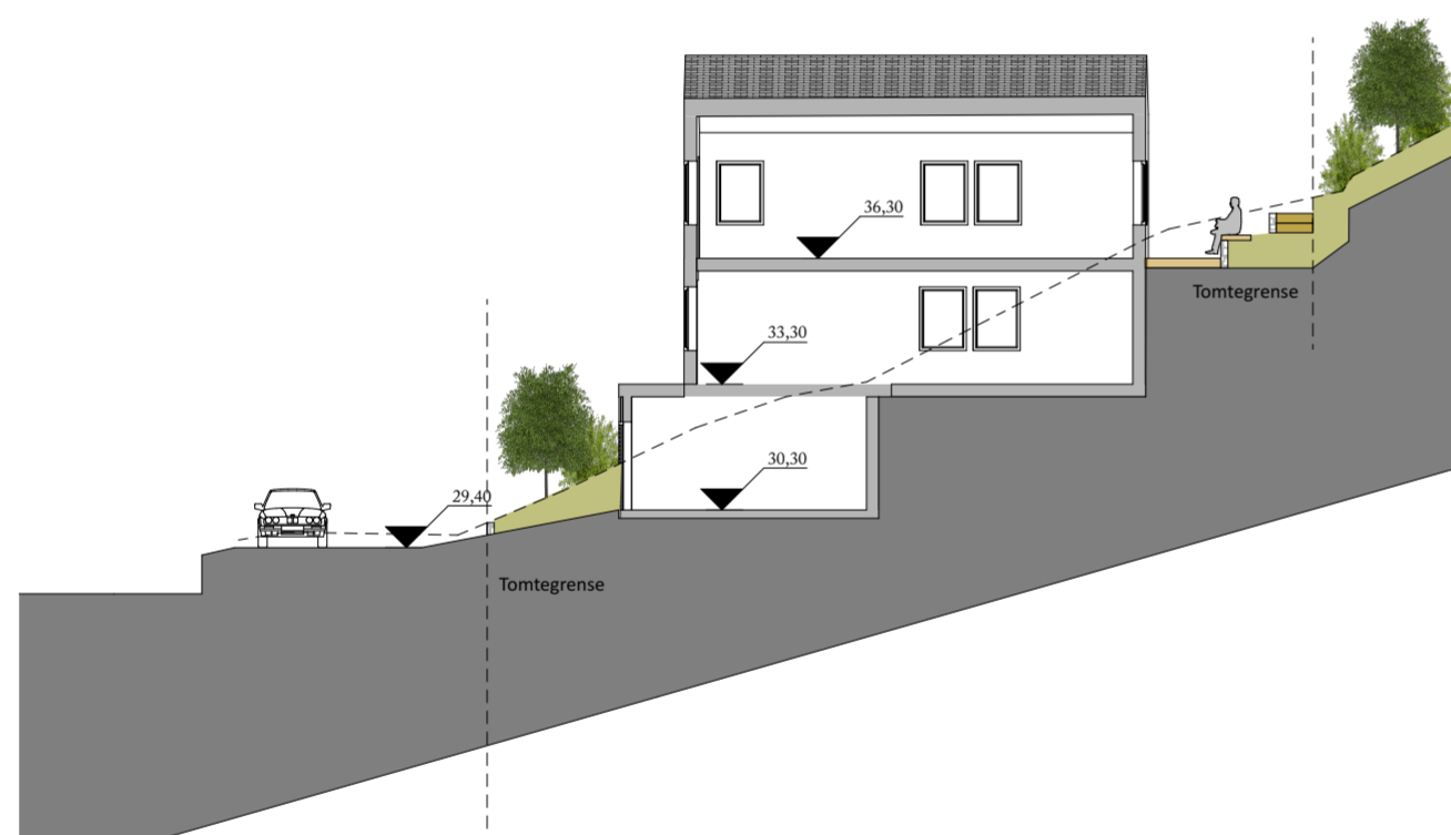
Snitt J-J gjennom felt B A2 mål 1:200
