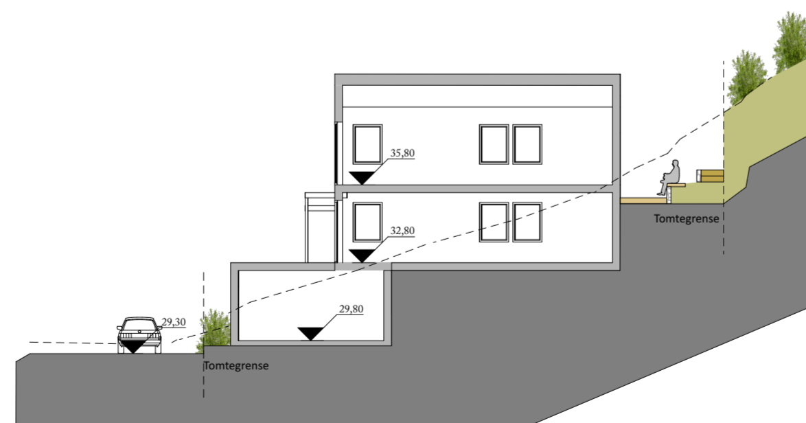
Snitt K-K gjennom felt B A2 mål 1:200
