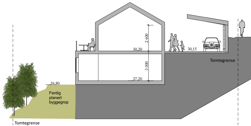
Snitt B-B Felt C A4 mål 1:100
