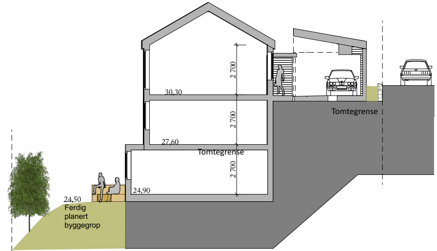
Snitt A-A Felt C A4 mål 1:100
