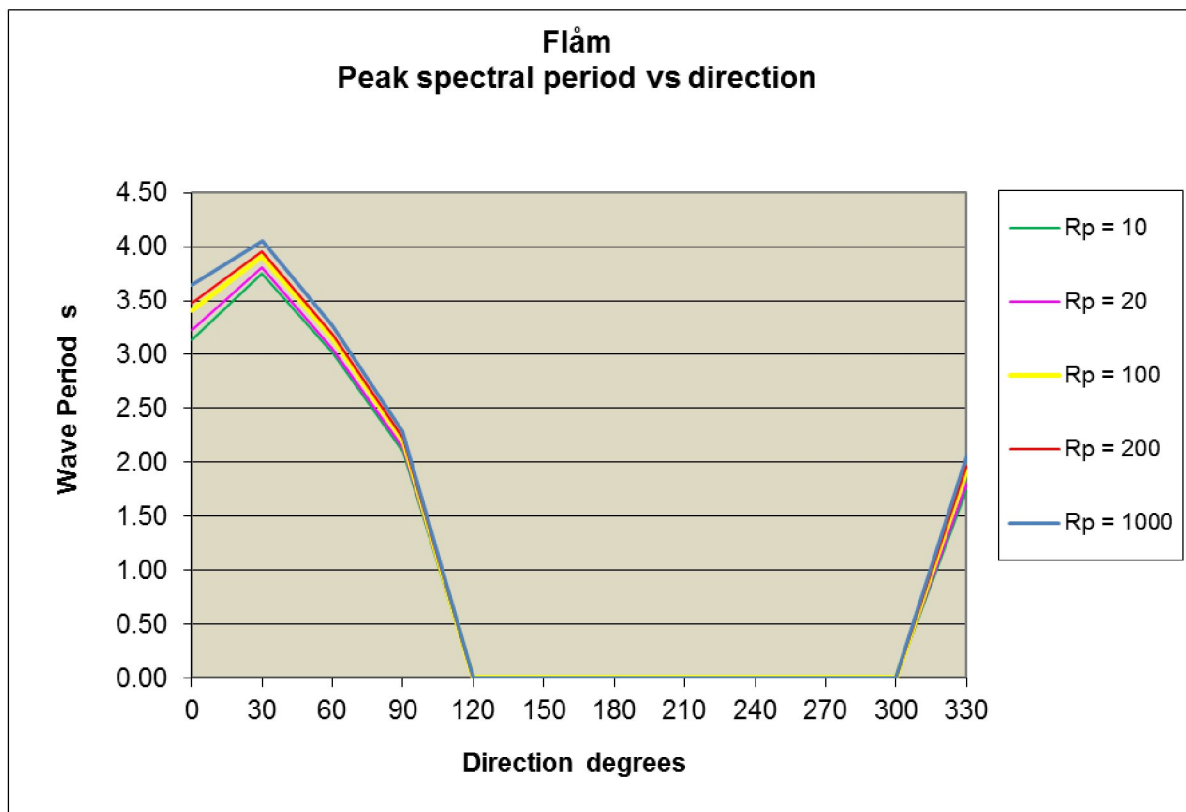
Figur 3 Ekstremverdier og returperioder av spektral topp-periode, T_p .
